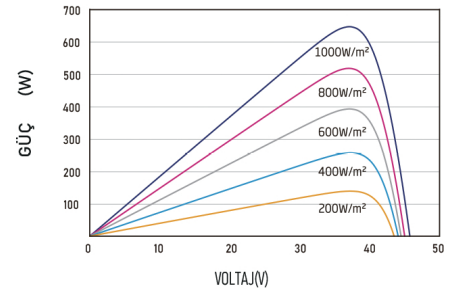
(P-V) GÜÇ - VOLTAJ EĞRİSİ
