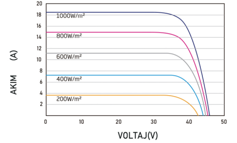
(I-V) AKIM-VOLTAJ EĞRİSİ
